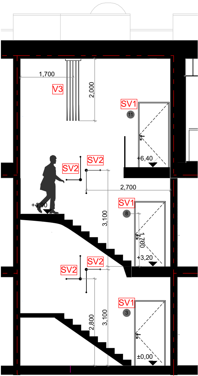
TREPI LÕIGE
